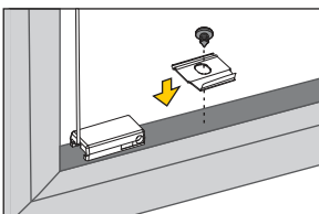
Halter am Glasfalz festschrauben
