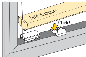
Sichtschutzprofil in Halter einrasten
