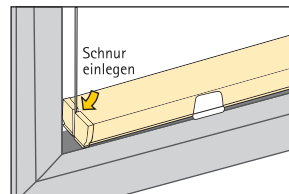
Schnur an der Seite des Sichtschutzprofils
